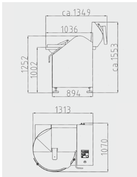
▲ ボウル容量70L、モーター22KW63A保護、インバータ22KW、重量1300kg
