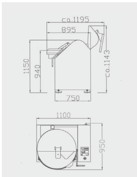
▲ ボウル容量50L、モーター11KW35A保護、インバータ15KW、重量730kg
